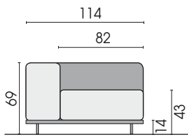
Frontansicht (Typ 208/254)
