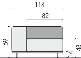
Seitenansicht (Typ 210/257)
