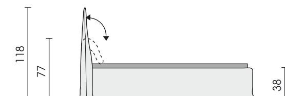
Seitenansicht
